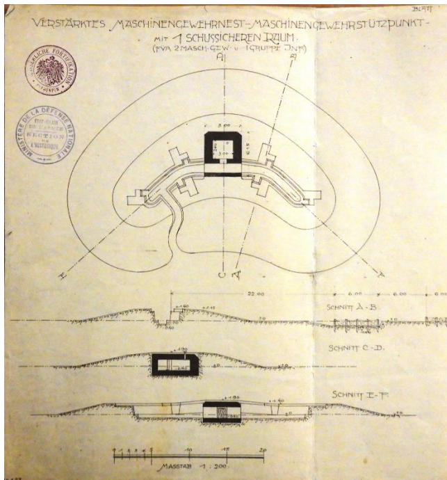
Opbouw van een mitrailleurstent met een bunker van het type II (Koninklijk Legermuseum, Fonds 185, doos 952).
