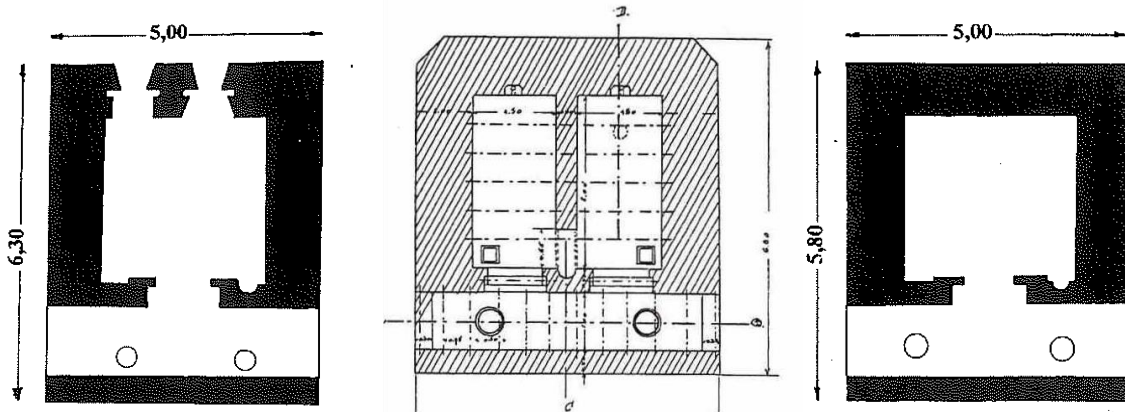
Grondplan van een MG type IV (links), een Masch. Gew. Stand zugl. Unterschlupf für 18 Man type I (midden) en een Masch. Gew. Unterstand type II (rechts) (© Simon Stevinstichting en GHEYLE W. & BOURGEOIS I. 2013, deel II, 202).
